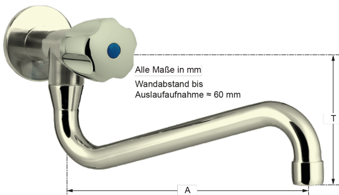
Wandanschluss 3/4"
