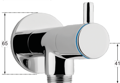
Abgang 3/4"
