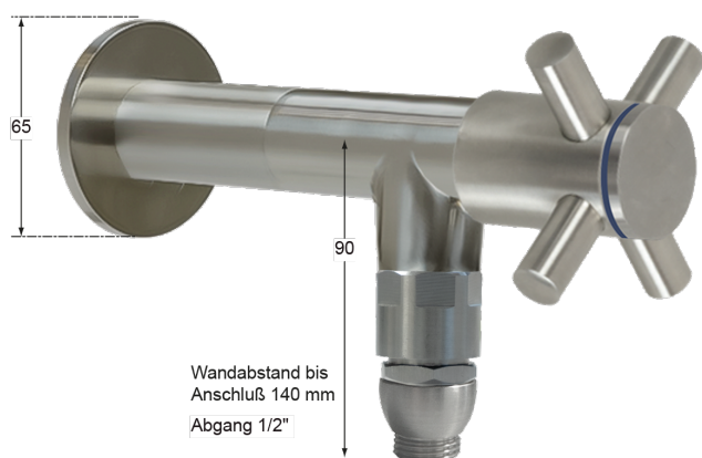
Wandanschluss 1/2"
