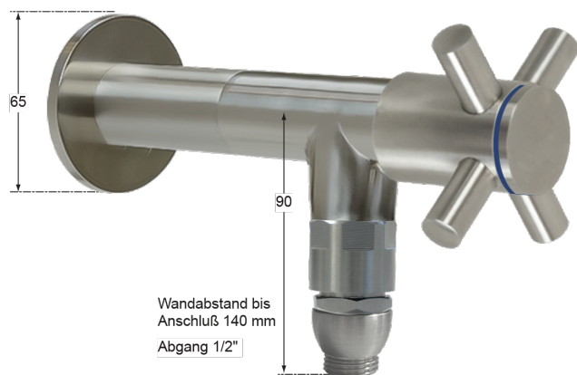
Wandanschluss 3/4"
