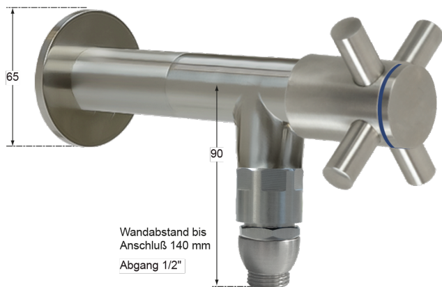
Wandanschluss 3/4"
