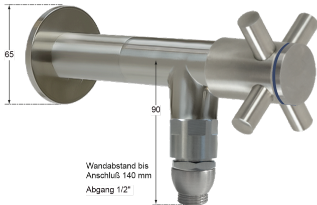
Wandanschluss 3/4"
