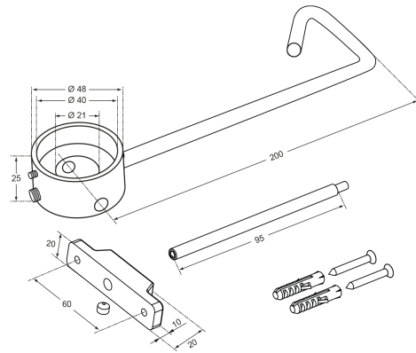
PA66 und komplett 1/2" EDELSTAHL
