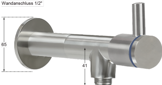
Wandanschluss 1/2"
