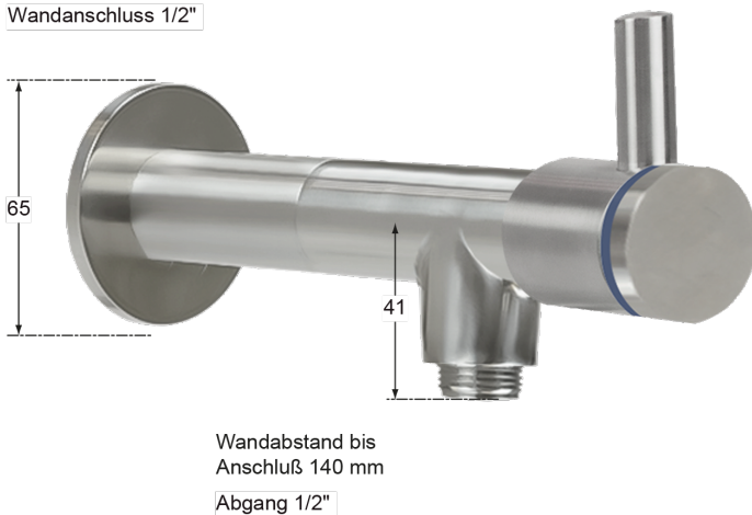
Wandanschluss 1/2"
