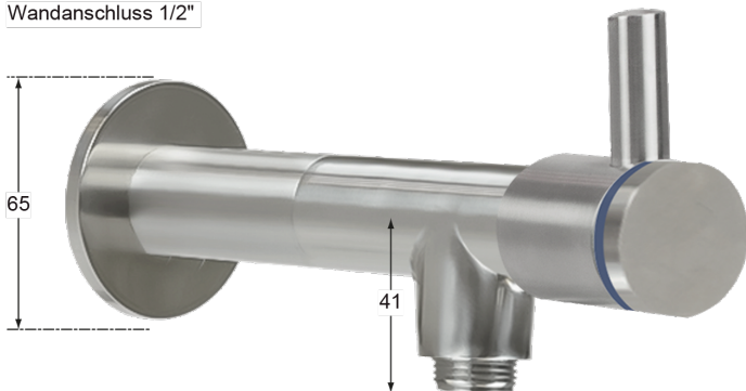
Wandanschluss 1/2"
