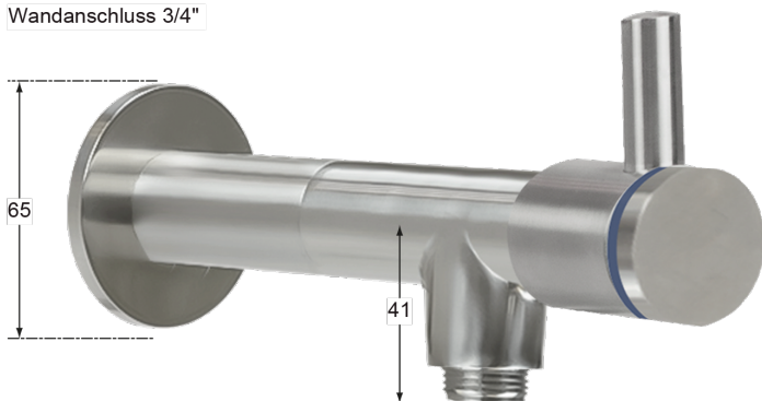
Wandanschluss 3/4"
