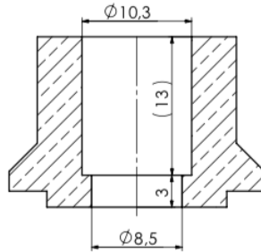
SCHNITT A-A
