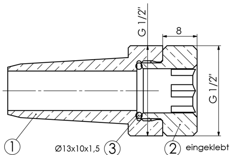
SCHNITT A-A
