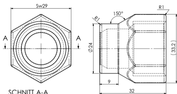
SCHNITT A-A MAßSTAB (3 : 1)
