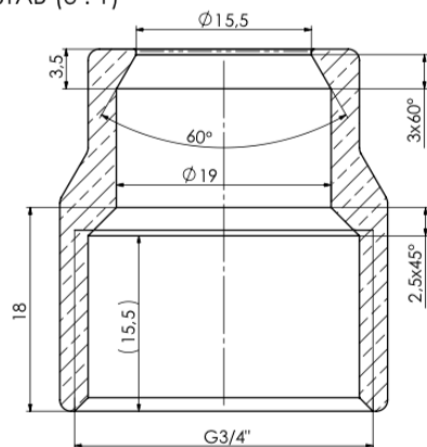
SCHNITT A-A MAßSTAB (3 : 1)
